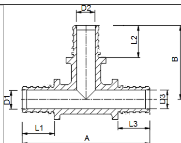
Тройник аксиальный/переходной
