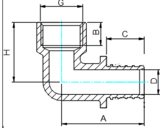
Угольник аксиальный ВР
