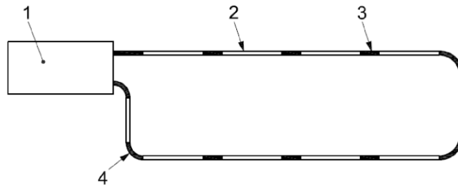
Рисунок 2 – Схема испытаний материала труб и фитингов PVC-C тип I на стойкость к аварийной температуре T_{авар}
